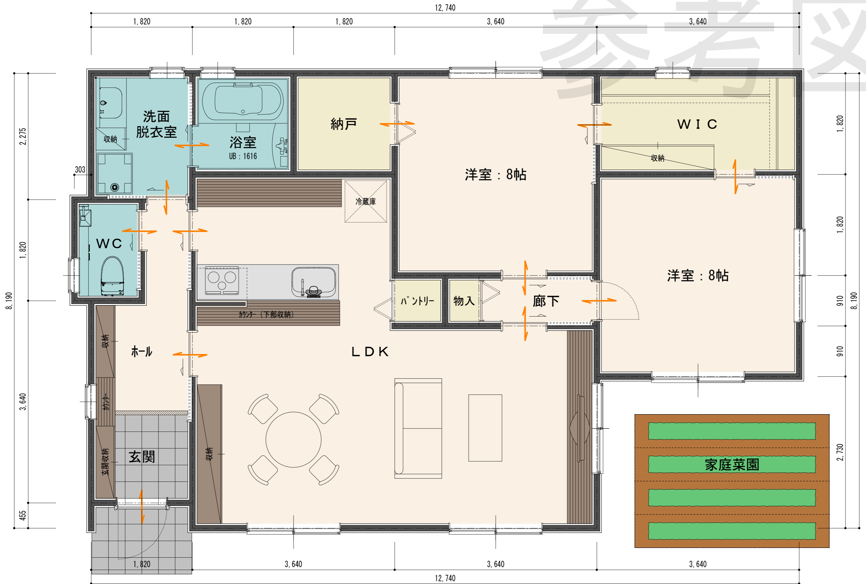
1階平面図
